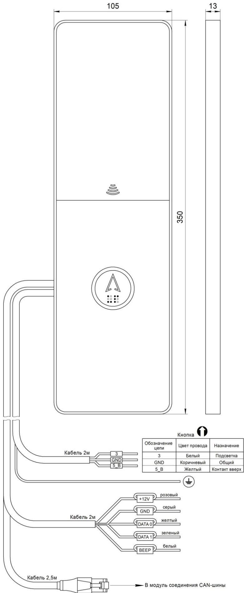
Рис.1 Внешний вид, габаритные и установочные размеры Вызывного поста МАЛАХИТ (жгут RJ45) НШЕК.468381.015-09
